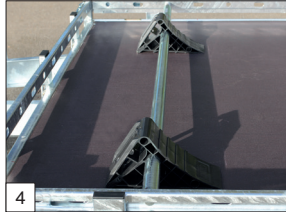
Optie: verstelbare wielblokkering model Combi Protect Rail, incl. 2x zwarte verschuifbare aanslag.
