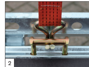
Standaard: voorzien van TÜV-goedgekeurde bindbeugels geïntegreerd in de zijrand, met een capaciteit van 1000 daN per stuk.
